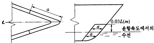
그림 3.5.1 충돌보호
