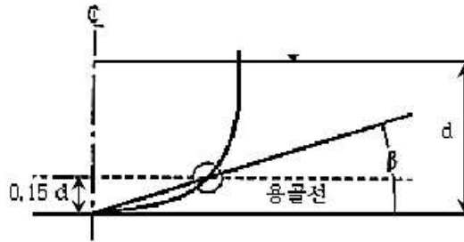
그림 3.2.4 등근 단면의 선저각도
