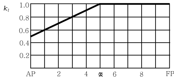
그림 3.2.3 길이방향의 슬래밍압력 분포계수 k_1
