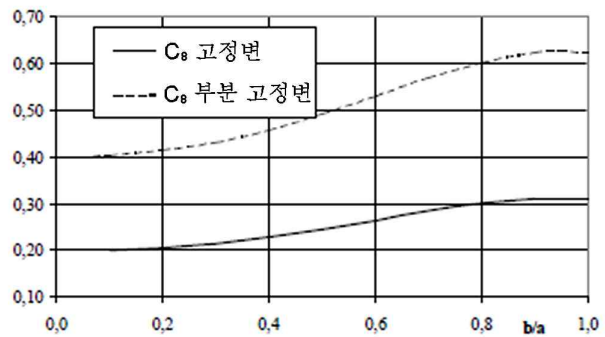
그림 3.5.8 계수 C_8
