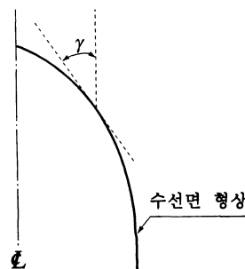
그림 3.2.6 각도 \gamma
