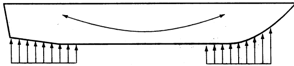
그림 3.2.10 선수미 파정 착수
