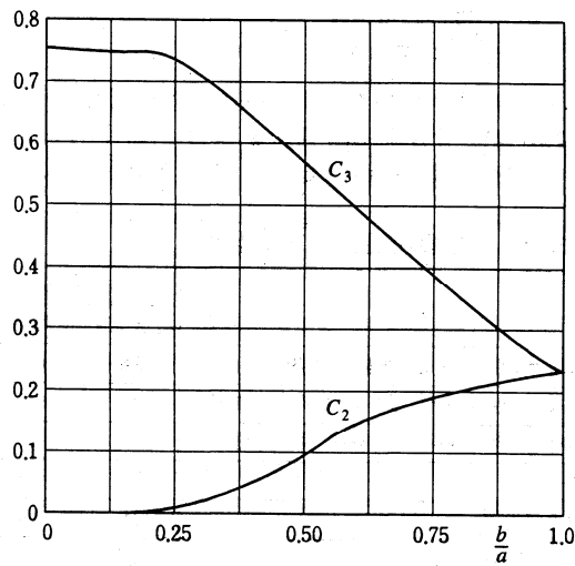
그림 3.5.4 계수 C_2 및 C_3
