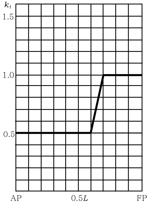
그림 3.2.7 쌍동선연결부 슬래밍 분포계수 k_t
